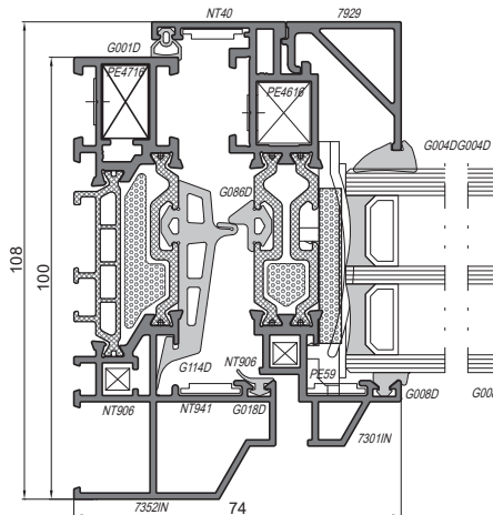
Ościeznica ze skrzydłem okiennym
