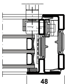
Vantail de fenêtre et cadre
