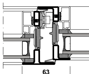
Vantail de fenêtre et vitrage fixe
